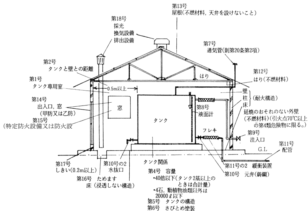
屋内タンク貯蔵所参考例
