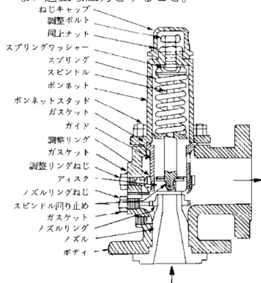
安全弁の構造例
