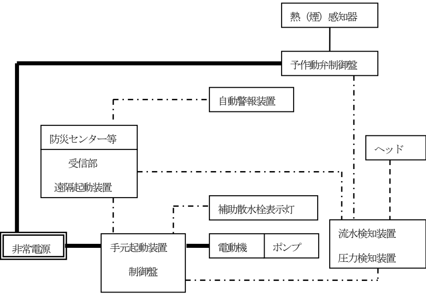
イ スプリンクラー設備、水噴霧消火設備及び泡消火設備の場合（第 37－16 図参照） 第 37－16 図
