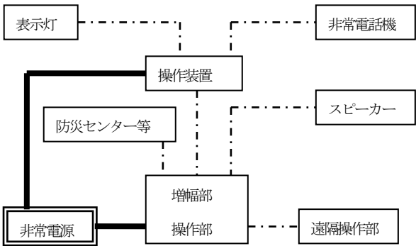
ク 放送設備の場合（第 37－22 図参照） 第 37－22 図
