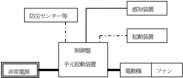
コ 排煙設備の場合（第 37－24 図参照） 第 37－24 図
