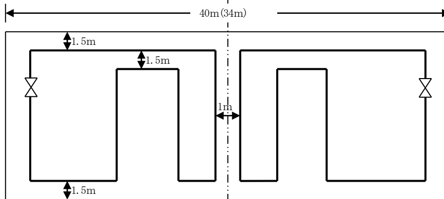
平面図
