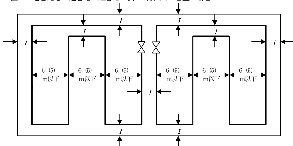
第24-68図 一边省略と二边省略の組合せの例2（特に広い居室の場合）
