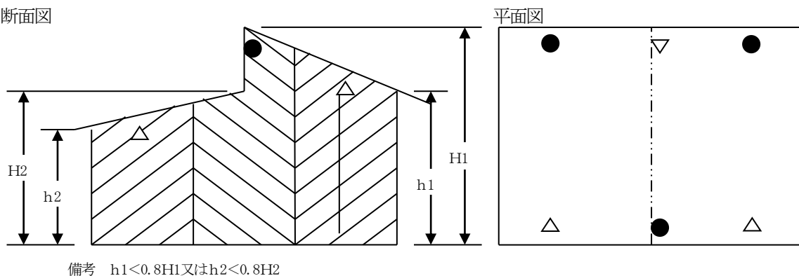
第24-101図 断面図
