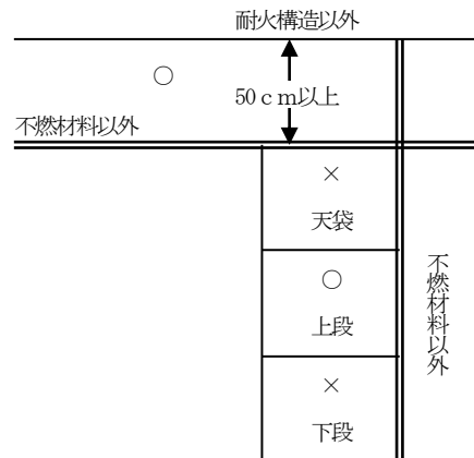
(イ) 押入等の壁が不燃材料以外のもの 第24-11図
