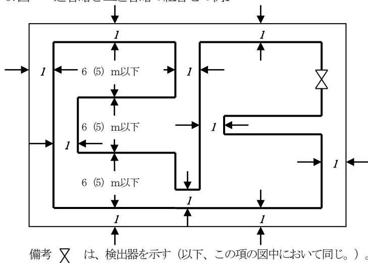
第24-67図 一边省略と二边省略の組合せの例1
