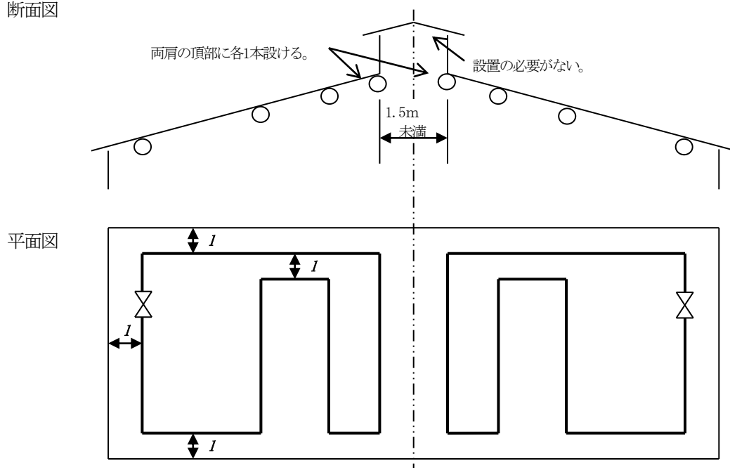
第24-88図 断面図
