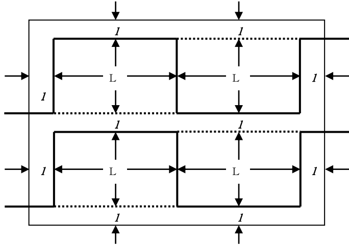
第24-64図 一辺省略の例2
