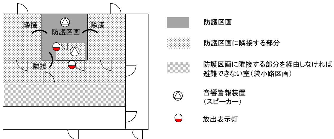
(消火剤が二酸化炭素で前室を設けた場合の一例)
