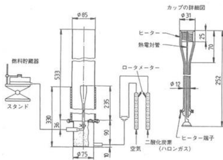
図1 カップ燃焼装置
