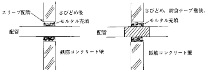
例図2 配管の固定装置の部分
