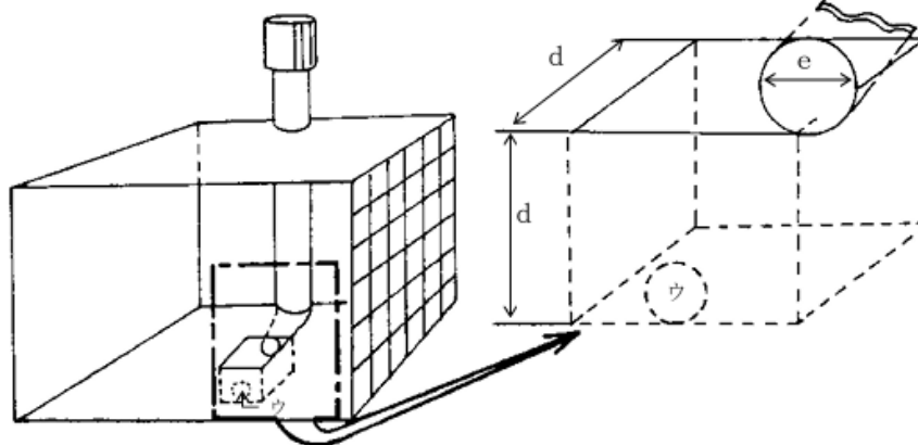
例図2 —ためますを整備室の中央に設ける場合の例—
